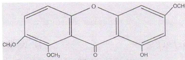
"C" Decussatin
